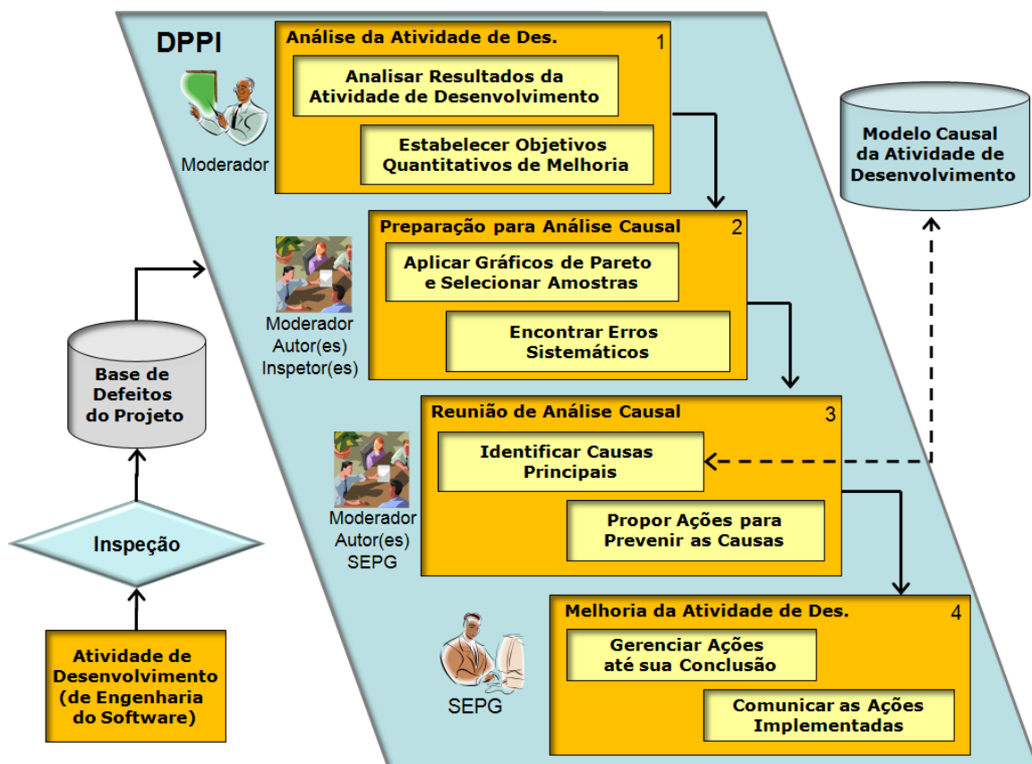
Figura 4.2. Visão Geral da Abordagem DPPI.
