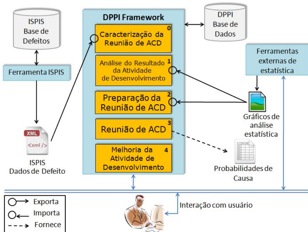
Figura 5.5. Arquitetura da Ferramenta DPPI Framework.
