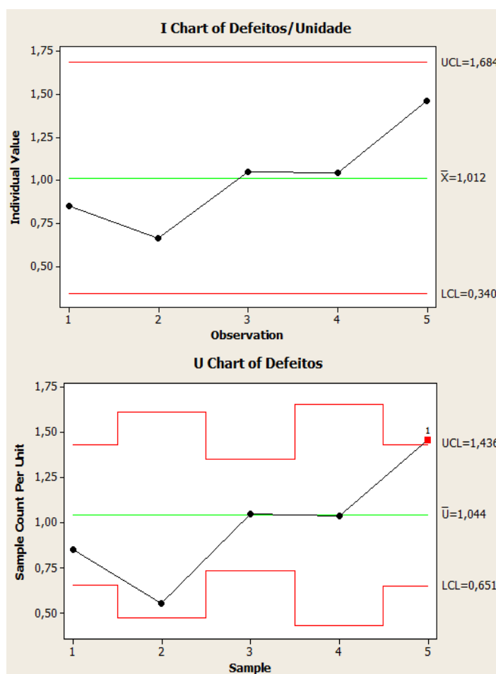
Figura 3.2. Gráficos XmR e U, Considerando Dados Equivalentes.
