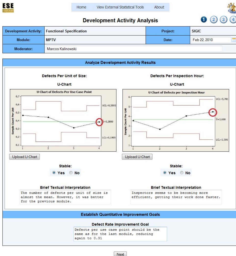
Figura 5.7. Apoio Ferramental à Atividade de Análise da Atividade de Desenvolvimento.
