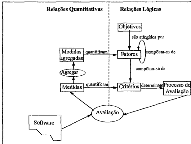
Figura IV.1: Modelo Rocha (ROCHA, 1983)
