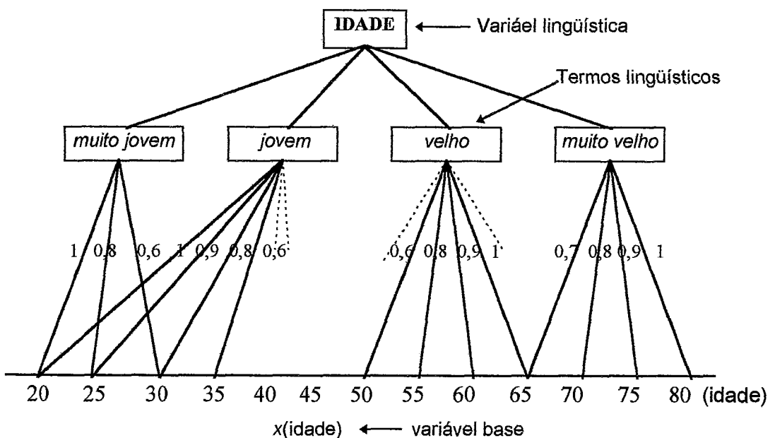
Figura III.3: Variável lingüística "Idade" (ZADEH, 1973b)
