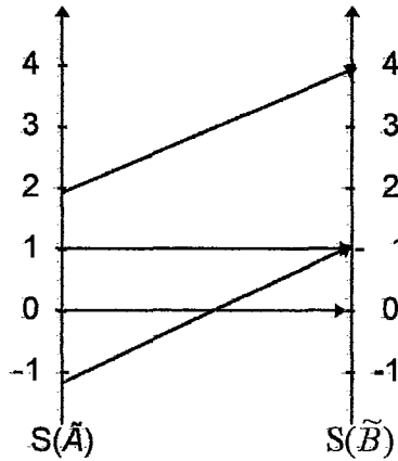
Figura III.1: O Princípio da Extensão (ZIMMERMANN, 1991)
