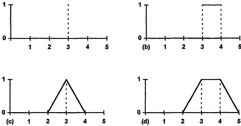
Figura III.2: Comparação de um número real e um intervalo nítido com um número fuzzy e um intervalo fuzzy respectivamente (KLIR et al. , 1995a)
