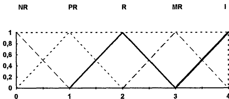
Figura VI.3: Funções de pertinência de números fuzzy, para termos lingüísticos
