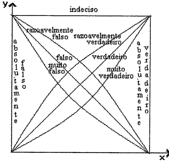
Figura III.4: Variável linguística “Verdade” (BALDWIN, 1979)
