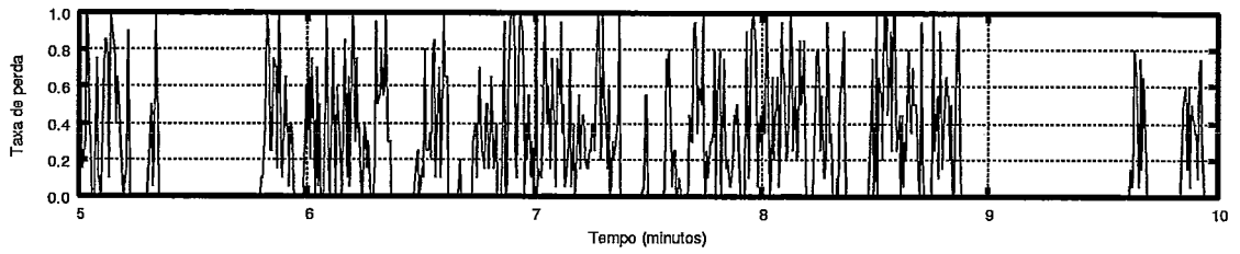
(a) Taxa de perda com alta variabilidade em um cenário simulado com tráfego de fundo MMPP
