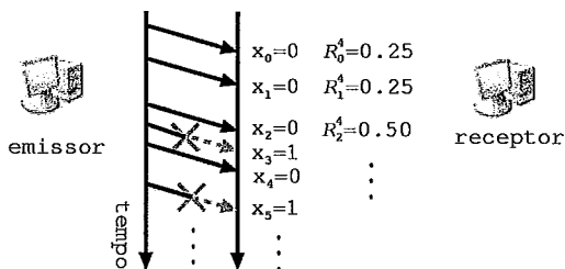
Figura 3.2: Taxa de perda R_t^F
