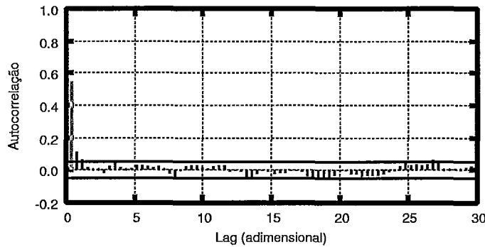
Figura 4.3: Autocorrelação da taxa de perda ( F = 20 ) para um modelo de perdas de Gilbert-Elliot simplificado com a fração de perda de 10% e rajadas de perdas média de 20 pacotes
